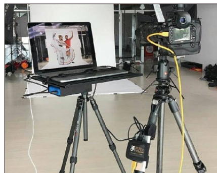
使用製品：テザーテーブルエアロマックブックプロ17インチ用(TTAM17BLK)、エアロセキュアストラップ(SS004)、エアロXDC(AXDOBK)、エアロプロパッドマックブックプロ17インチ用(PDMAC17-2) Photo by Mauricio Urena
