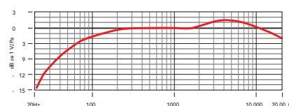
周波数特性
