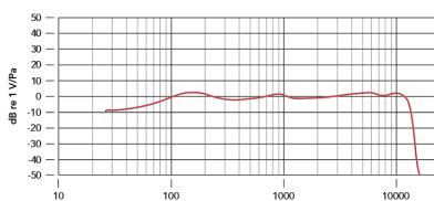
周波数特性
