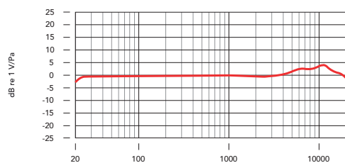
周波数特性
